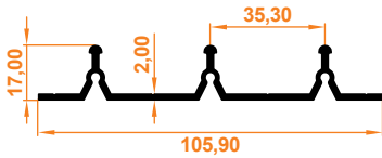
Üçlü Eşiksiz Alt Kasa Profil Triple Lower Case Profile Thresholdless
